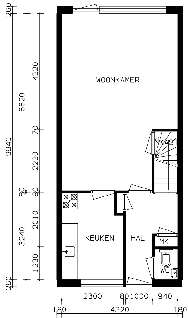
BEGANE GROND
